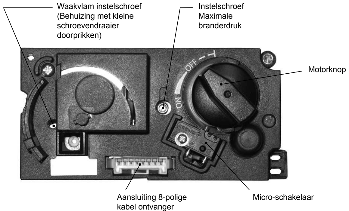
Figuur 24: Gasregelblok - Voorzijde
