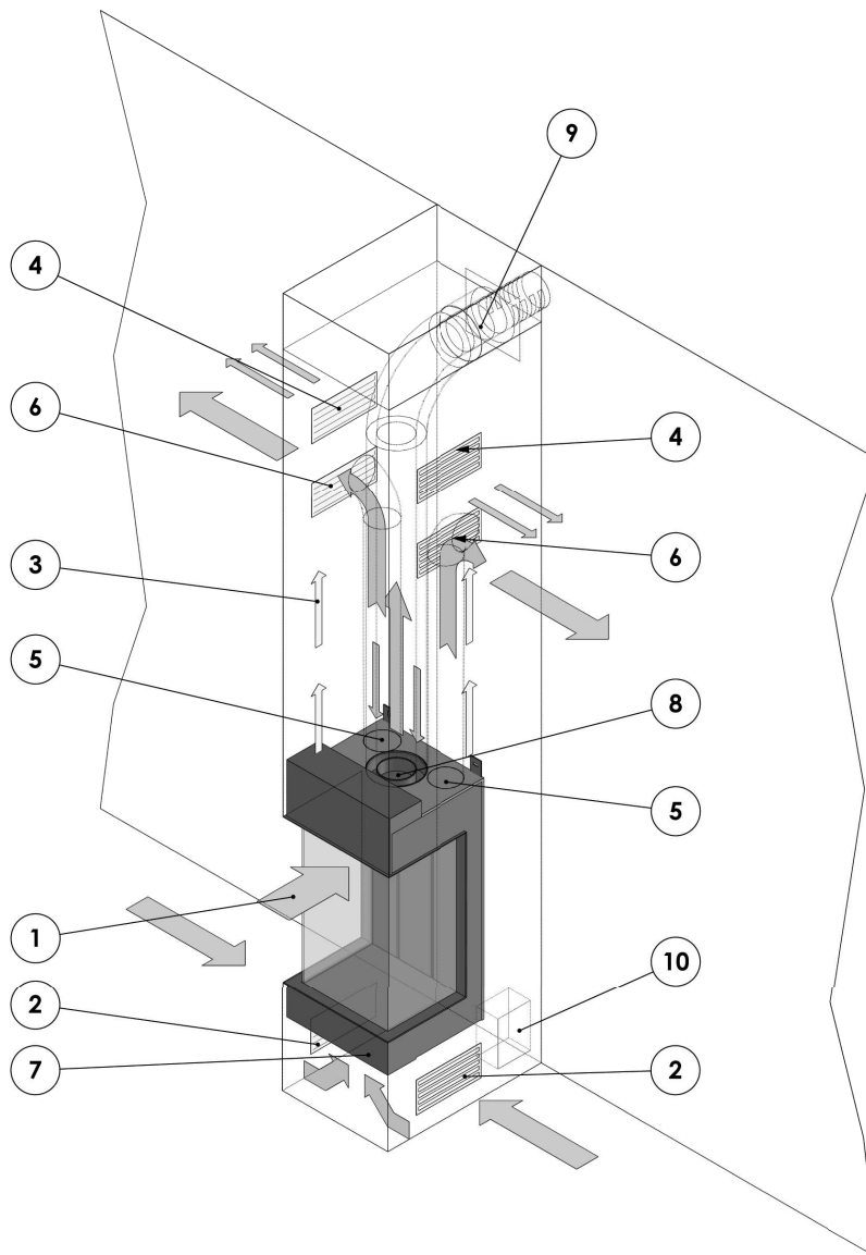
Figuur 16: INBOUW-HAARD: Toestel ingebouwd in geventileerde schouw Horizontale uitmondning van de rookgasafvoer/verbrandingslucht- toevoer via de muur. Voorzien van de opties/accessoires: • convectiepakket (= convectiemantel en 1x convectieset)
